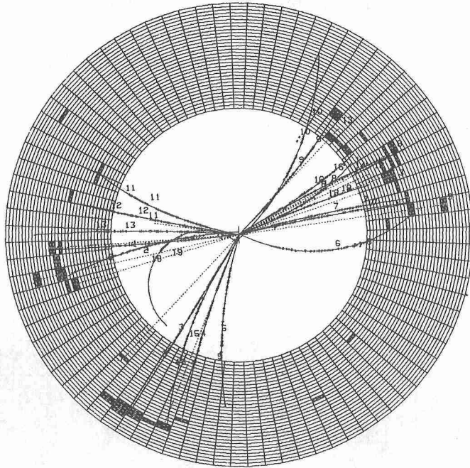
JADE 測定器で検出された、3つの Jet を示す反応。 左上の第3 Jet がグルーオンのこわれたものと思われる。 曲線は磁場中の荷電粒子の軌跡、黒い柵目は東大チームの 作った3000ケのシャーカウンターのうち光子等が当りエ ネルギーの測定されたカウンターを示す。
